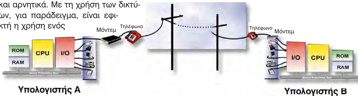
Σχήμα 3.8 Διασύνδεση υπολογιστών
